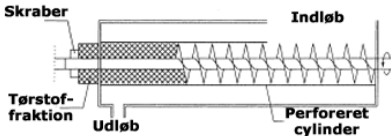
Figur 1. Principskitse af en skruepresse.
