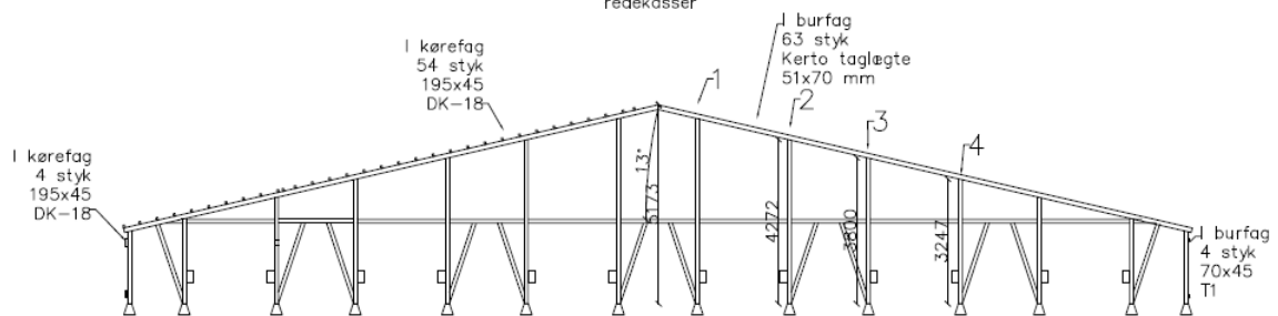
Snit A-A
