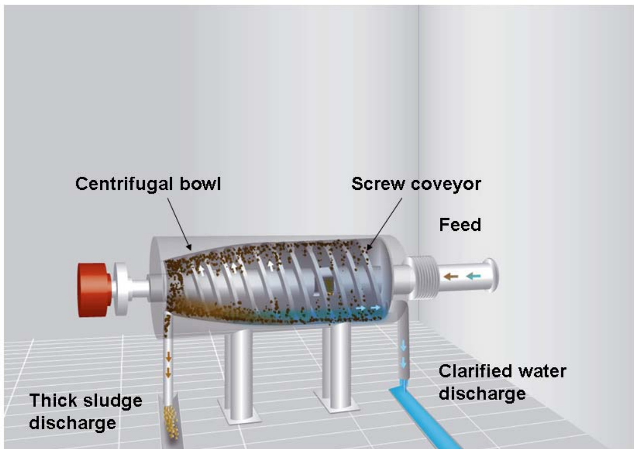
Figur 1. Principskitse af en dekantercentrifuge.
