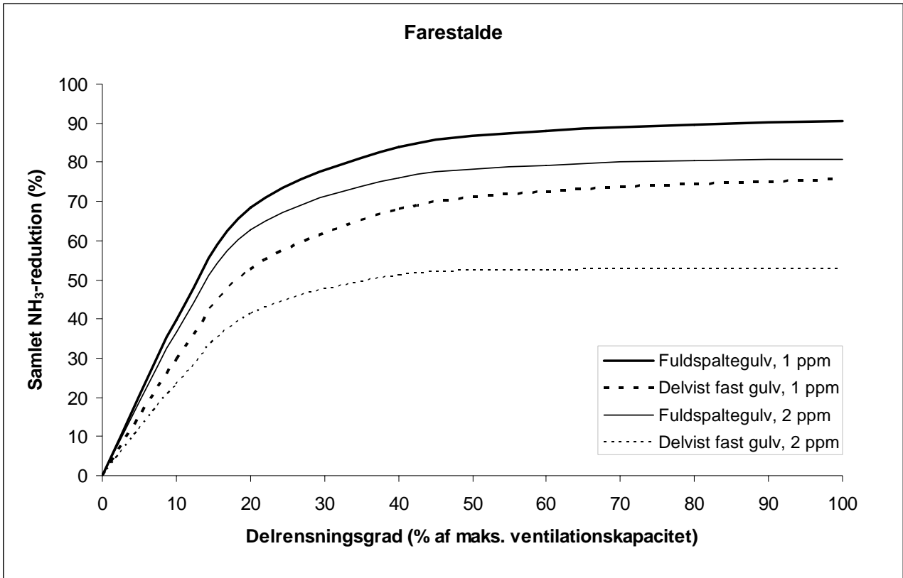
Figur 4. Sammenhæng mellem procentdel af maksimal ventilationskapacitet, der passerer en luftrenser i en farestald, og den årlige reduktion i ammoniakemission for en renser, der er i stand til at reducere ned til en given ammoniakkoncentration i ppm. Sammenhængen er vist for henholdsvis fuldspaltegulv og delvist fast gulv.
