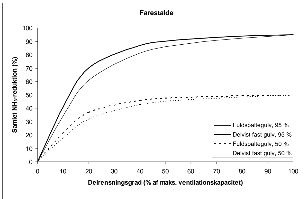
Figur 5. Sammenhæng mellem procentdel af maksimal ventilationskapacitet, der passerer en luftrenser i en farestalde og den årlige reduktion i ammoniakemission for en renser med en given renseeffekt i procent. Sammenhængen er vist for henholdsvis fuldspaltegulv og delvist fast gulv.
